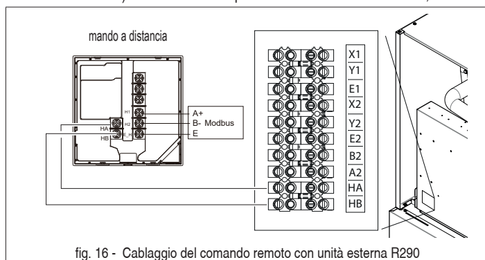
fig. 16 - Cablaggio del comando remoto con unità esterna R290
