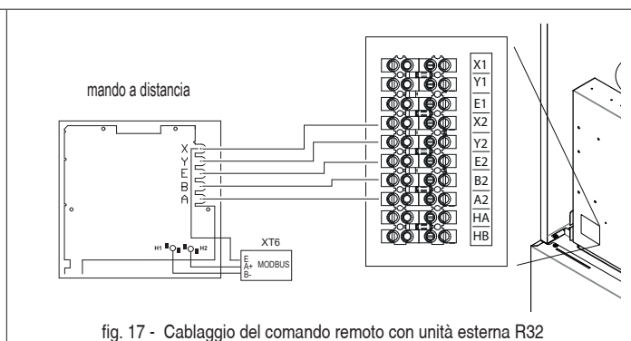
fig. 17 - Cablaggio del comando remoto con unità esterna R32
