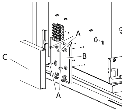
fig. 18 - Instalación del control remoto
